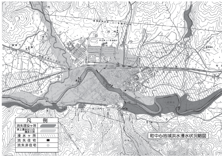
▲羽越水害時の町中心地域洪水浸水状況略図
