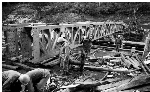
▲玉川口地内中の橋の工事の様子
