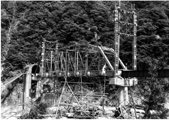
▲玉川第4鉄橋復旧工事
